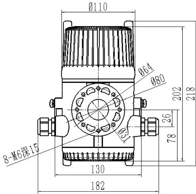
图 6.1a MBP-1 壳外型尺寸图
