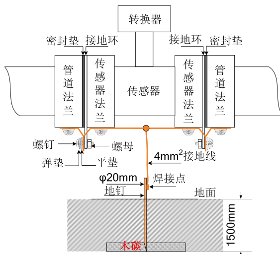
图 1.3 转换器接地示意图
